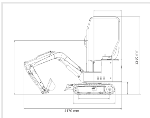
Dimensões principais
